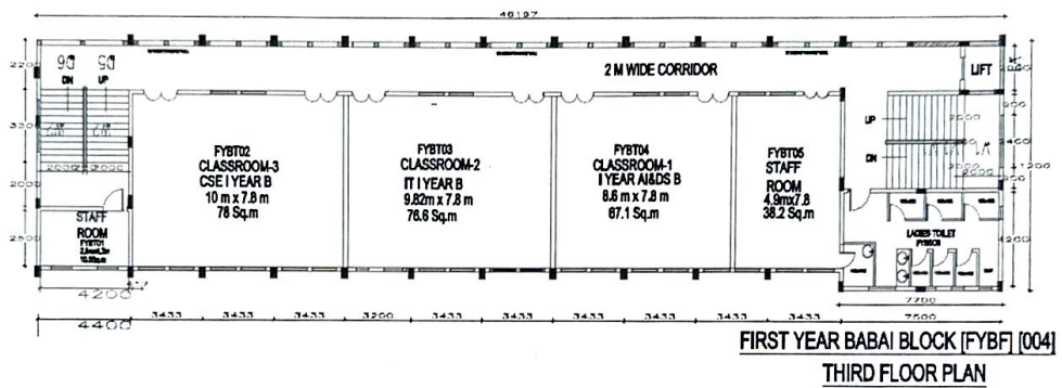
DR. K. S. BABAI BLOCK - THIRD FLOOR PLAN
