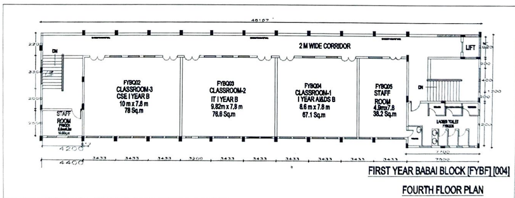
DR. K. S. BABAI BLOCK - FOURTH FLOOR PLAN
