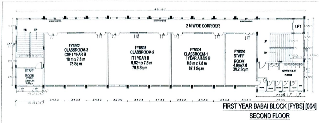
DR. K. S. BABAI BLOCK - SECOND FLOOR PLAN
